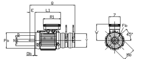
Крепеж у основания ВЗ размерностью 160-280
