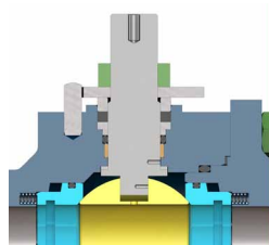
Исполнение управляющей цапфы и соединения корпуса с крышкой для температур до 200 °C
