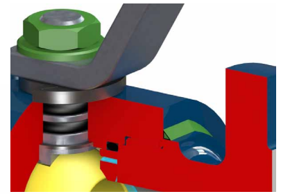
ЦЕЛЬНОСВАРНОЙ КОРПУС
