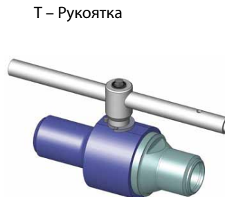
T – Рукоятка
